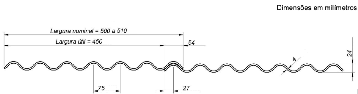
Figura 1 – Perfil da telha-padrão ondulada PO, largura 0,50 m
